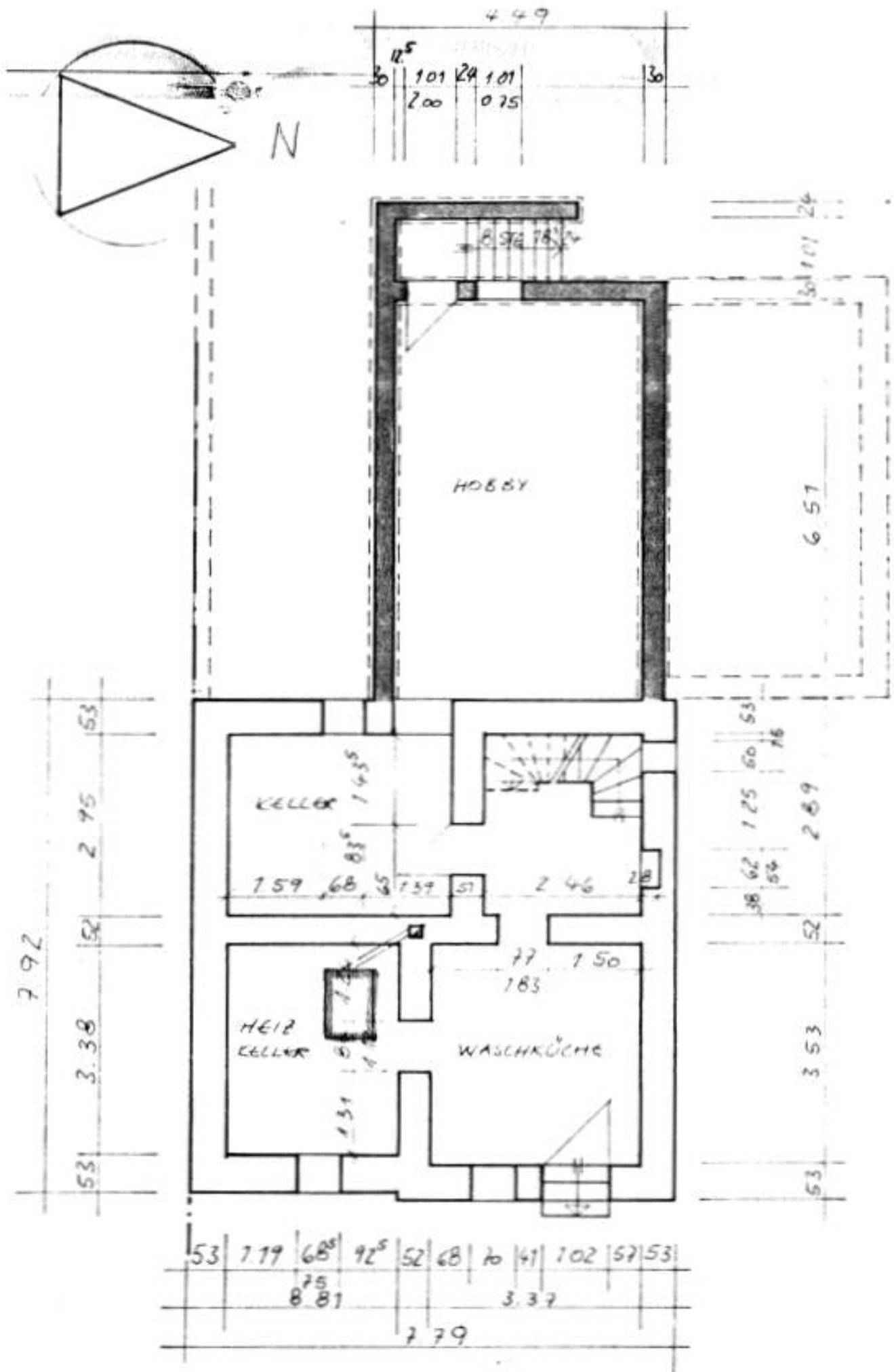
KELLERGESCHOSS
