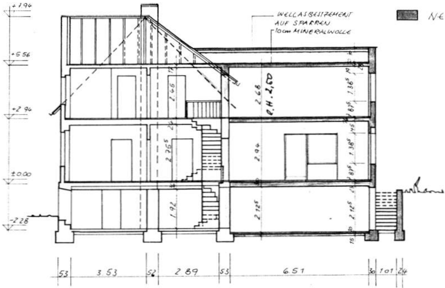
SCHNITT
